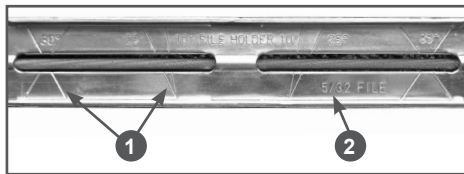
Рис.17 Обойма напильника
