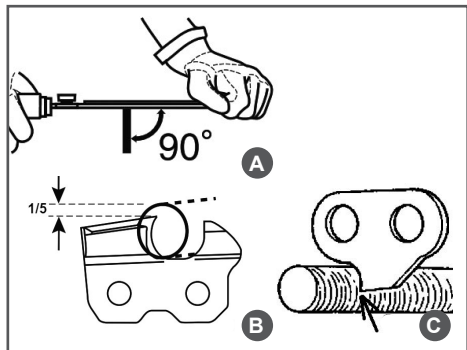
Рис.19 Заточка цепи
